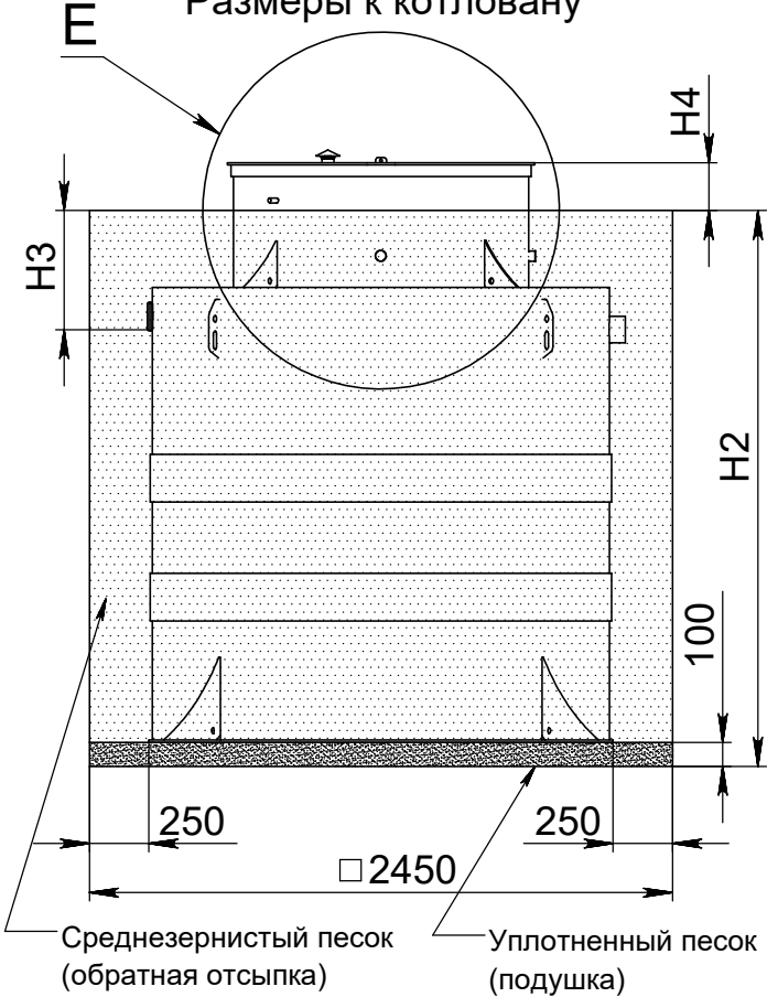
Размеры к котловану
