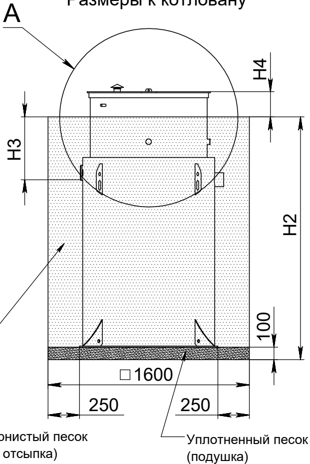
Размеры к котловану
