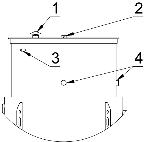
A (1 : 20)
